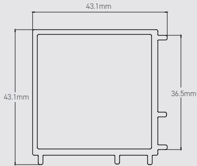
Corner Post A-08169
